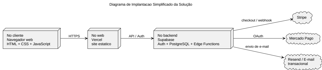
Figura 11 – Diagrama de implantação simplificado da solução
