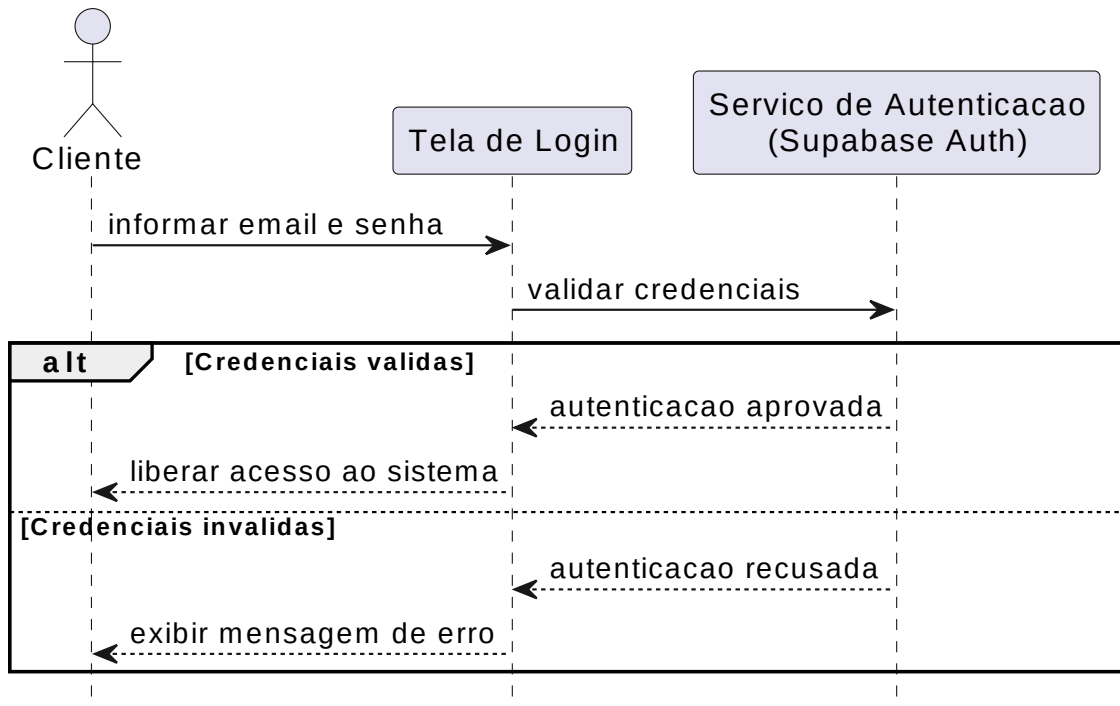
Figura 6 – Diagrama de sequência do caso de uso Autenticar usuário
