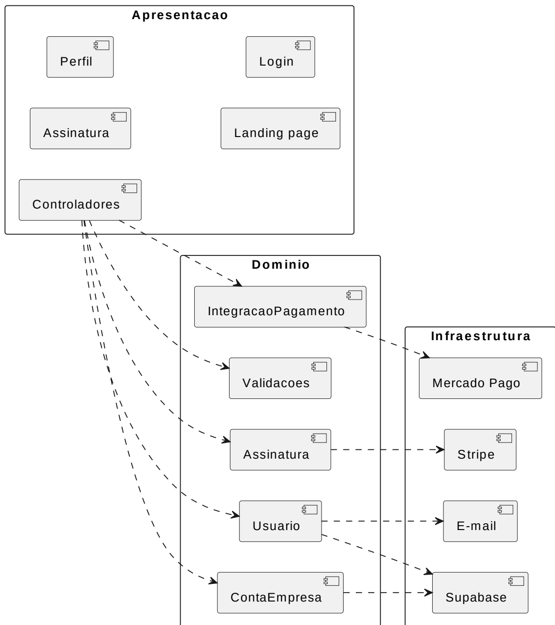
Figura 10 – Diagrama de pacotes da arquitetura lógica
