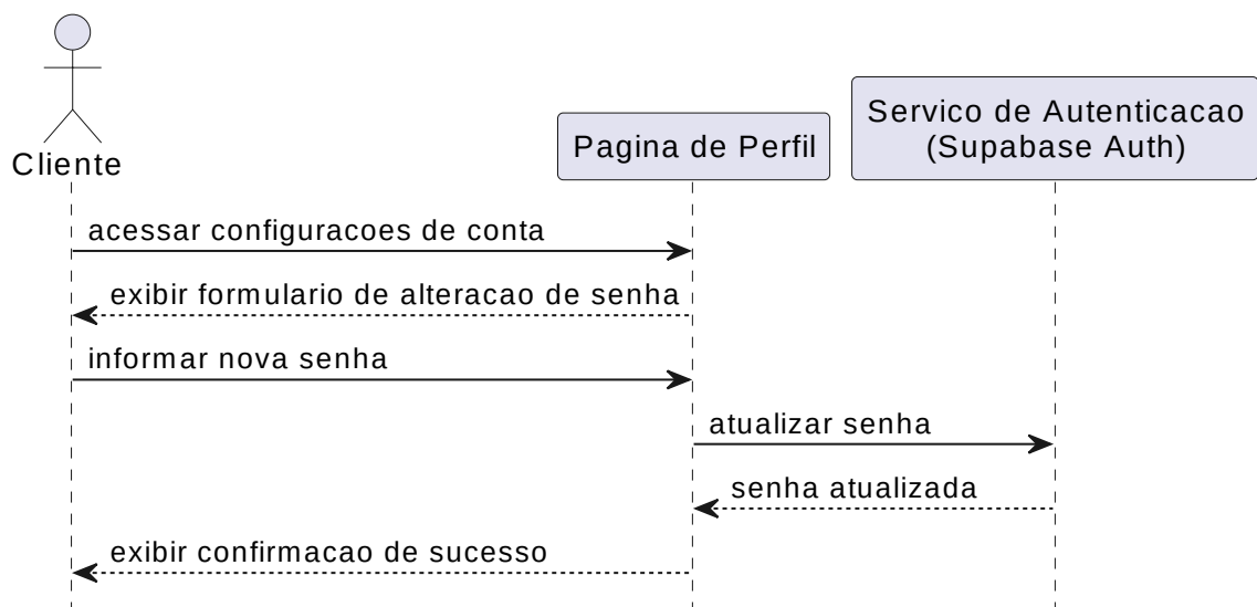
Figura 7 – Diagrama de sequência do caso de uso Alterar senha
